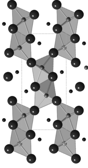
Goethite
