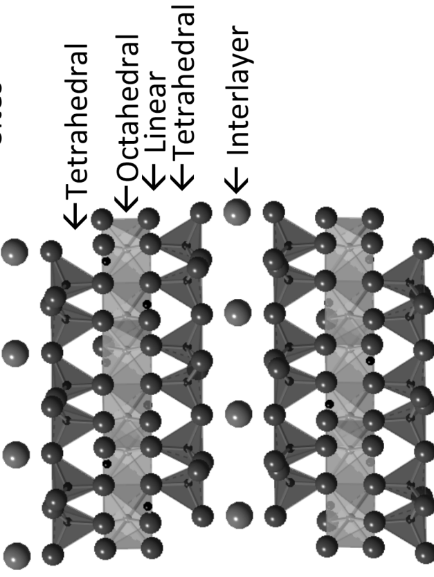
Muscovite
