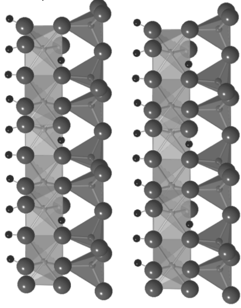
Kaolinite (Kaolin Group)
